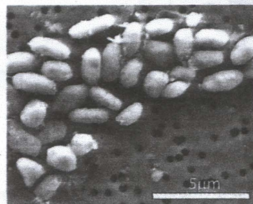
Bakterien GFAJ-1 hittades i en sjö i Kalifornien.
